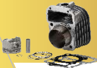
KIT CILINDRO DE MOTOR COMPLETO C/ JUNTA E ANEL CG 125 TITAN 02/08 // CG 125 FAN 125 05/08 // NXR 125 BROS 03/05 COD. 12003
